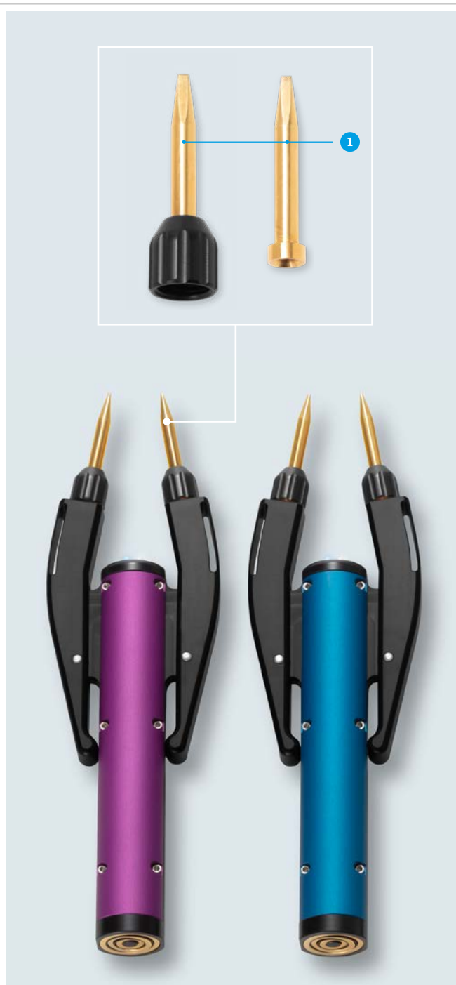
1 Pozlacený hrot vyměnitelných pinzet
